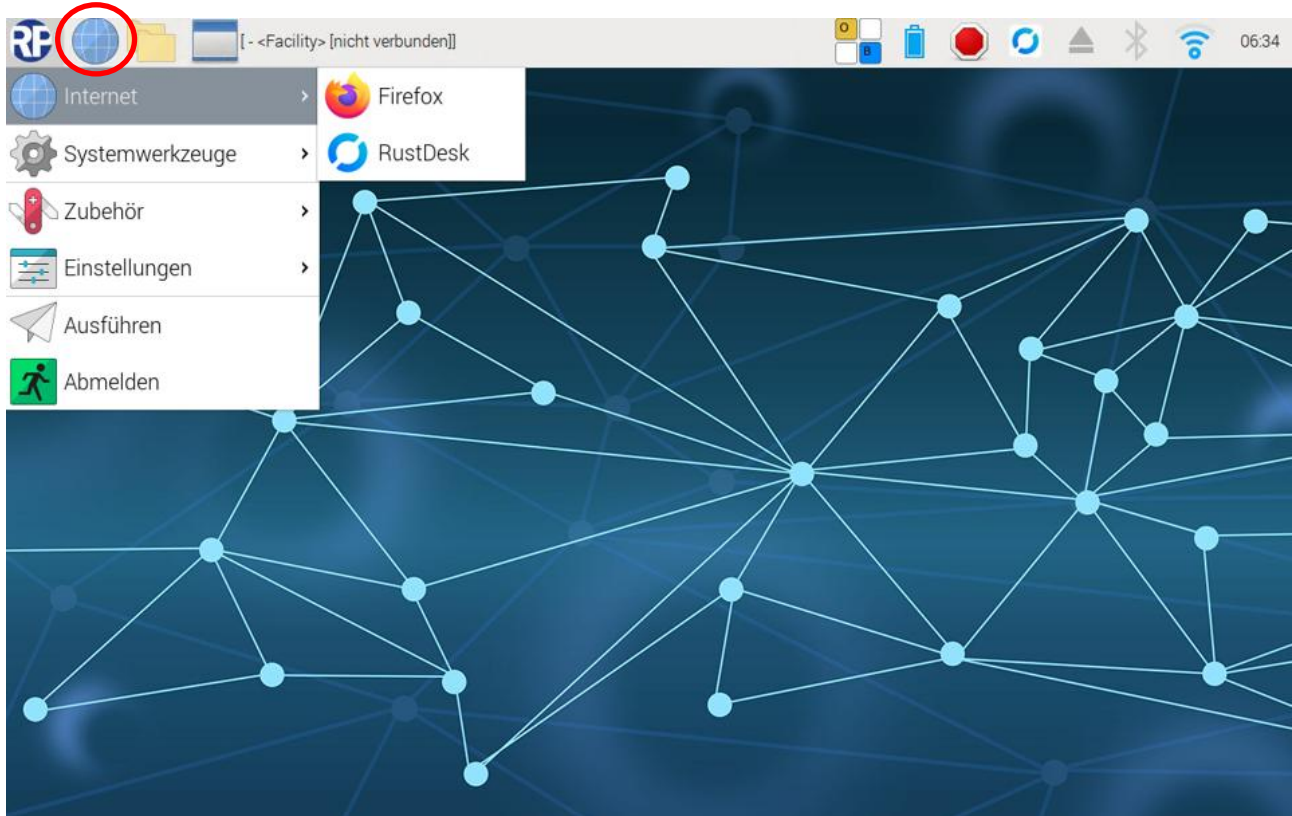
Abbildung 96 Startmenü -> Internet
