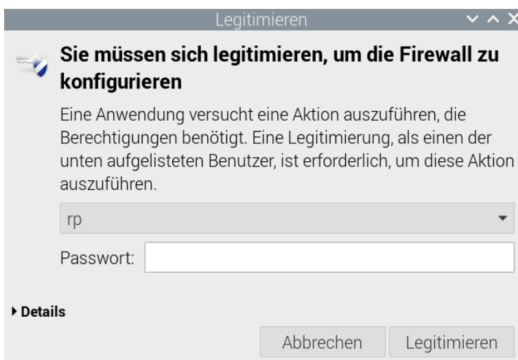
Abbildung 115 Firewall Legitimierung
