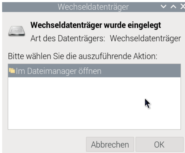
Abbildung 89 Speichermedium bestätigen
