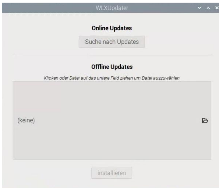
Abbildung 106 WLXUpdater
