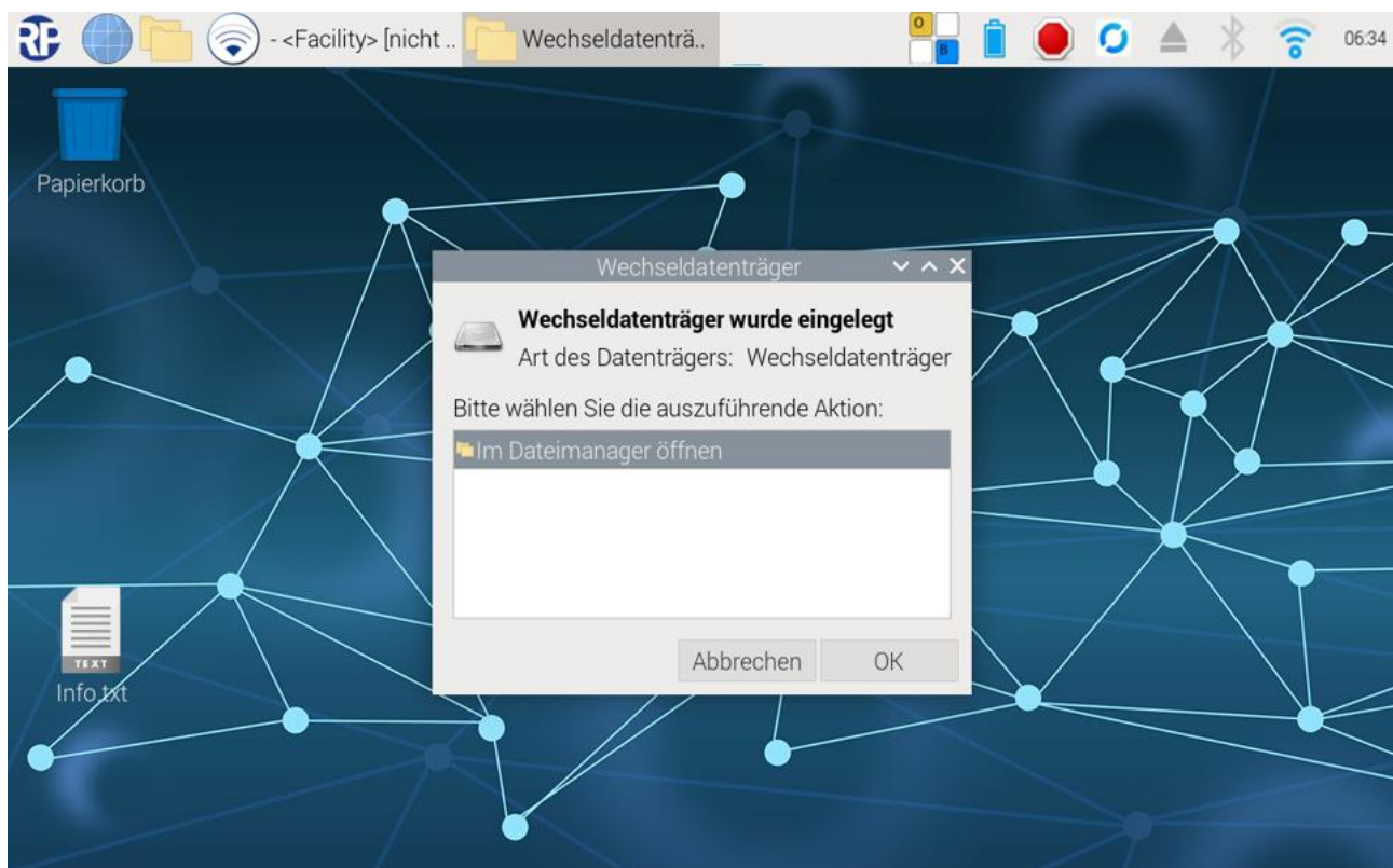
Abbildung 74 Speichermedium bestätigen
