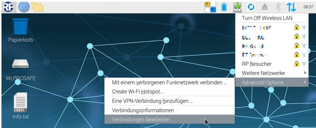
Abbildung 49 Verbindungen bearbeiten
