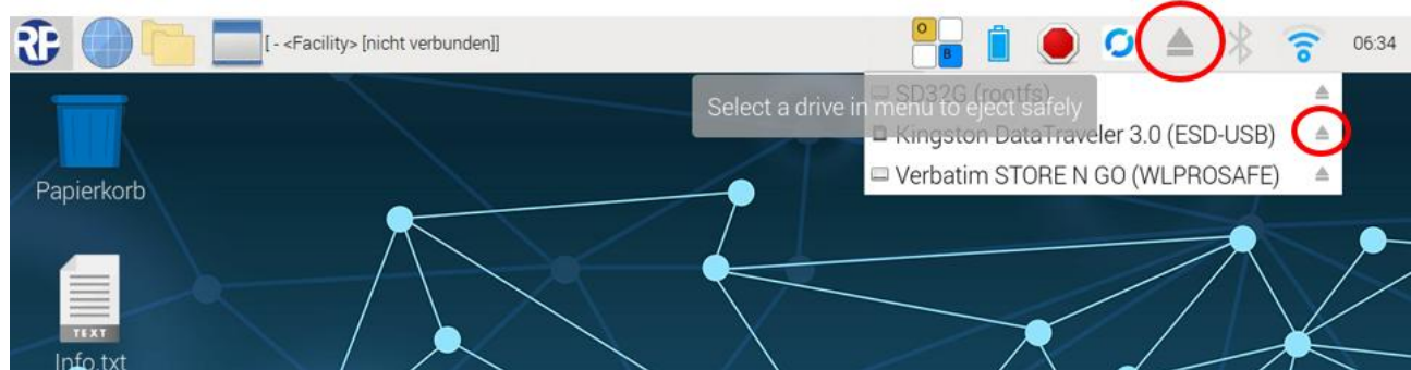
Abbildung 80 Speichermedium auswerfen
