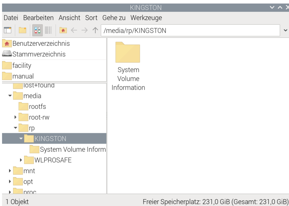
Abbildung 19 Speichermedium Dateiexplorer-Ansicht
