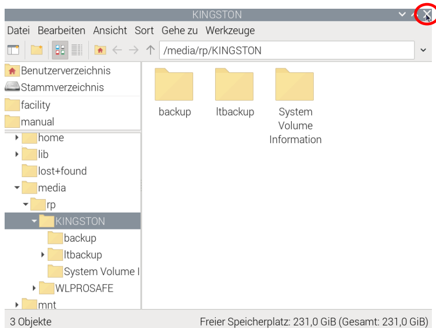
Abbildung 79 Dateexplorer schließen
