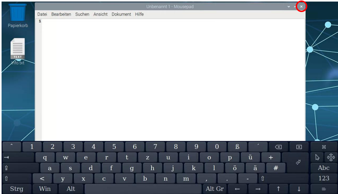
Abbildung 102 Texteditor schliessen
