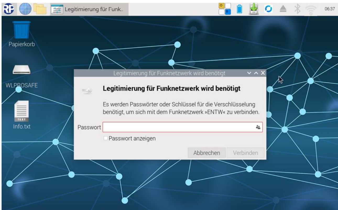
Abbildung 55 WLAN-Schlüssel eingeben
