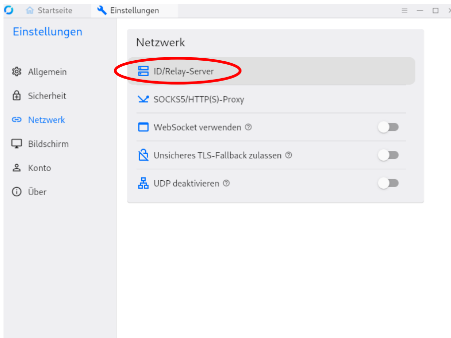
Abbildung 70 Rustdesk ID/Relay-Server
