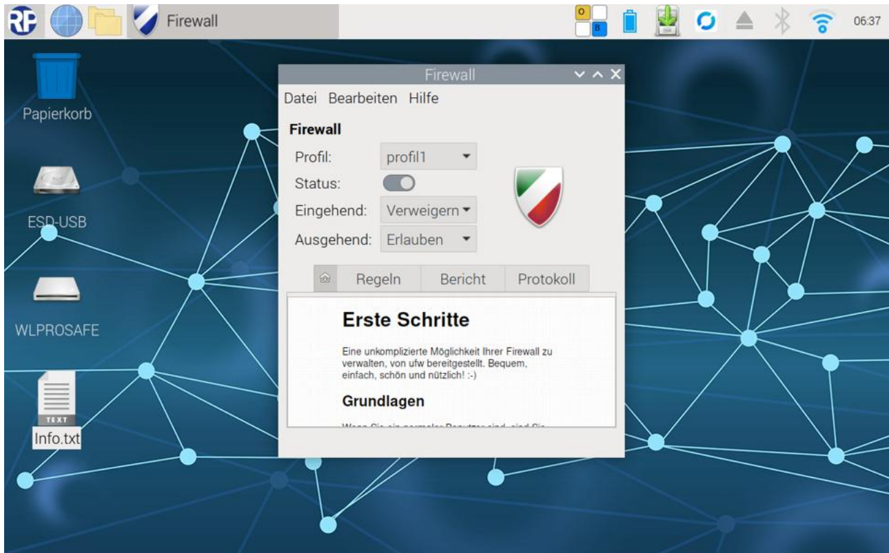
Abbildung 116 Firewall Fenster
