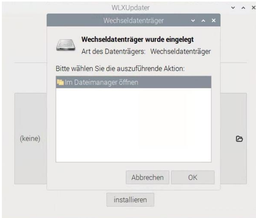
Abbildung 110 Speichermedium bestätigen
