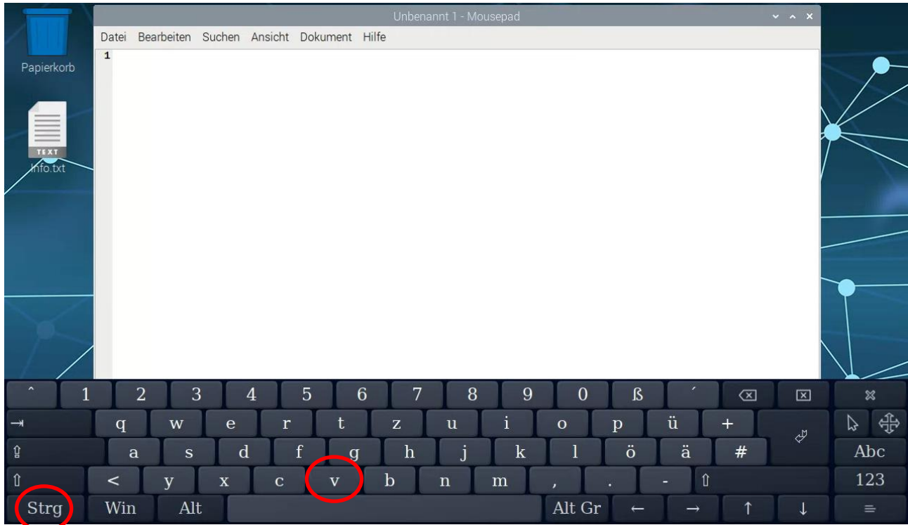
Abbildung 98 Texteditor
