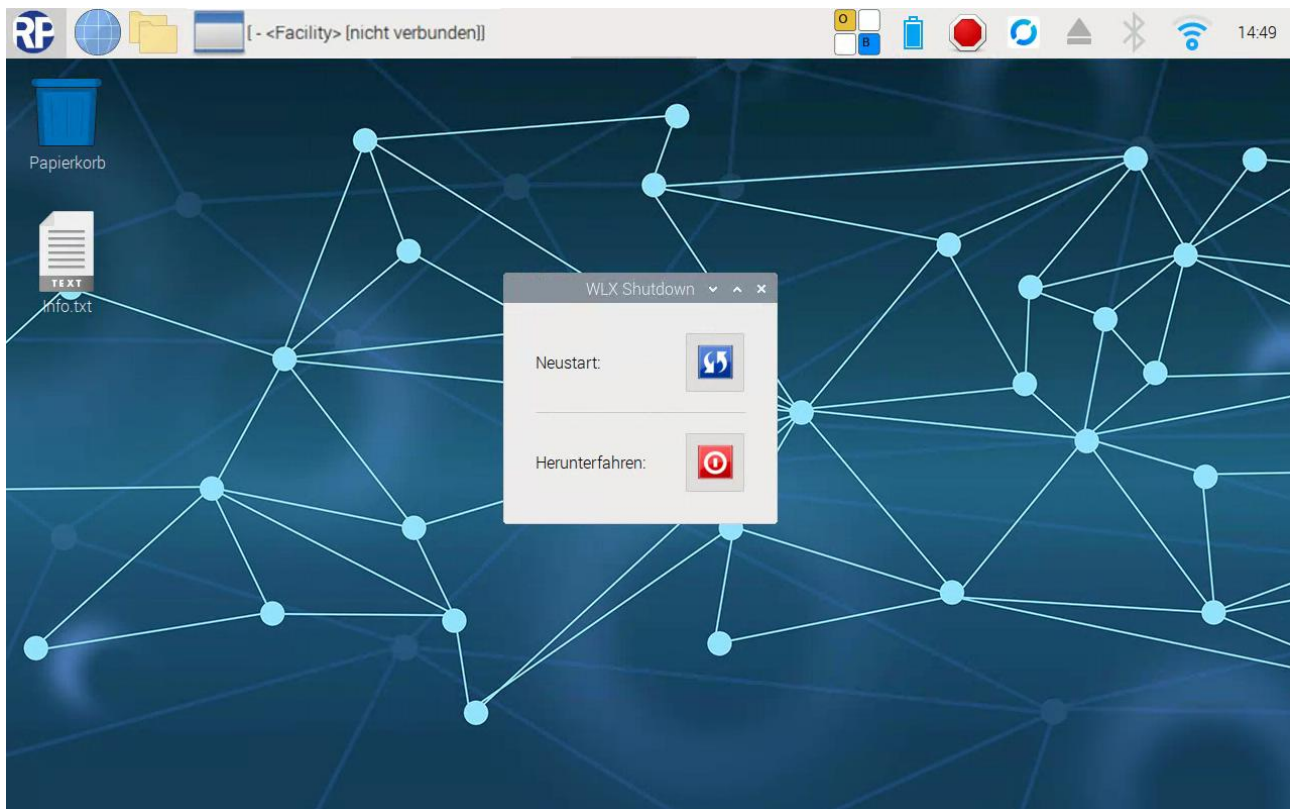
Abbildung 12 WLX Shutdown
