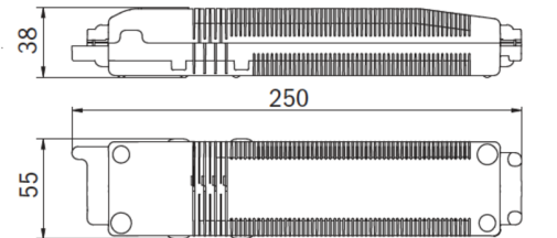
Einzelbatterie-Elektronik-Box (UH-1)
