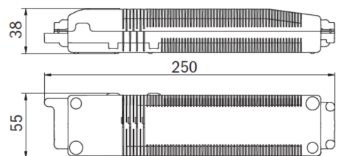
Einzelbatterie-Elektronik-Box (UH-1)
