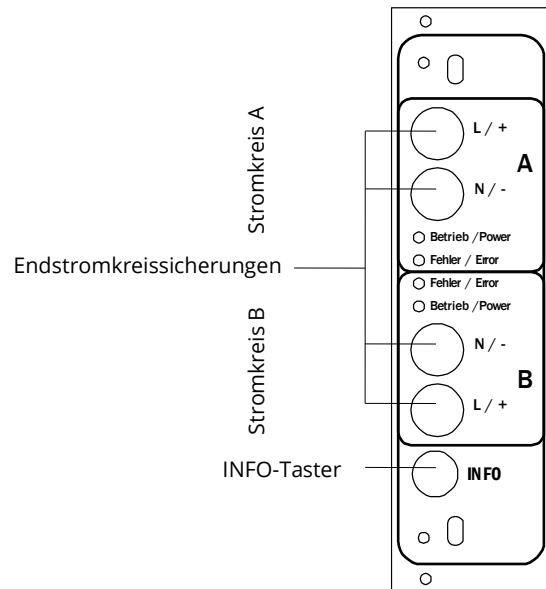
Abbildung 17: Stromkreismodul
