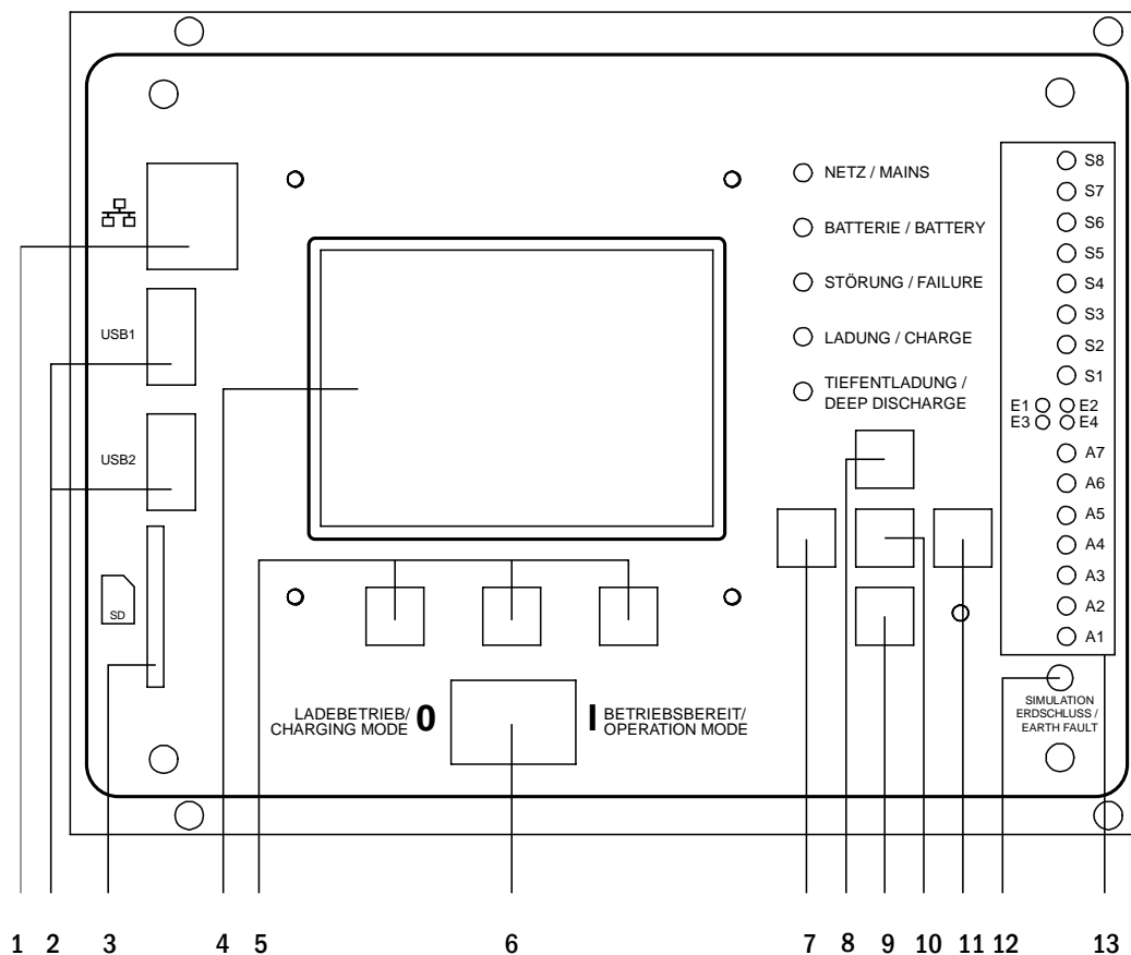
Abbildung 16: Zentrale Steuer- und Überwachungseinheit
