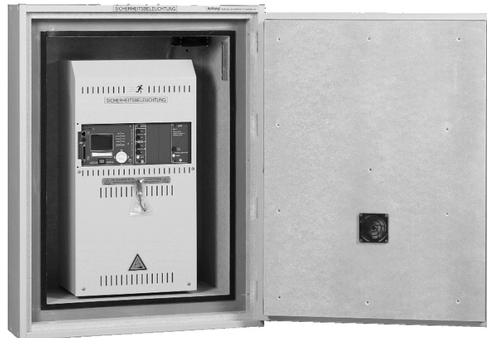
Abbildung 13: microControl plus im E30-Brandschutzverteilergehäuse
