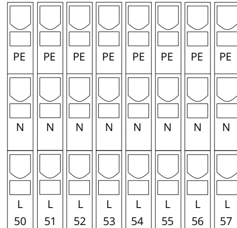
Abbildung 5: SAM-Eingänge
