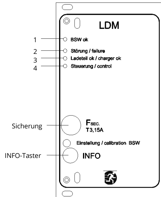
Abbildung 18: Lademodul LDM25
