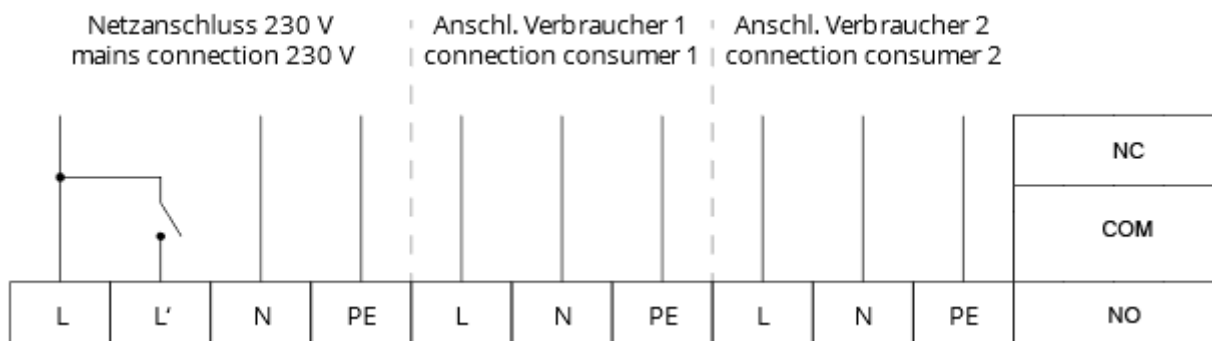
Abbildung 4: Anschlußplan NVG-RW
